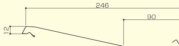
製品形状図 (働き幅228)
